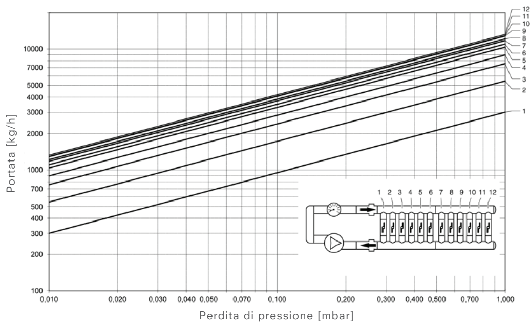
Diagramma perdite di carico collettore PLASTICLIMAZIONE
